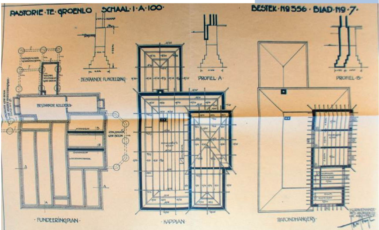
Constructietekening (bron ECAL)
