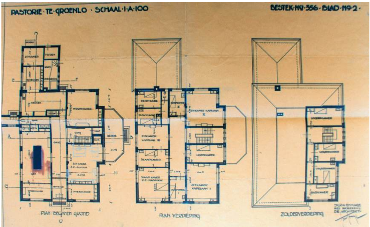
Ontwerp plattegronden (bron ECAL)
