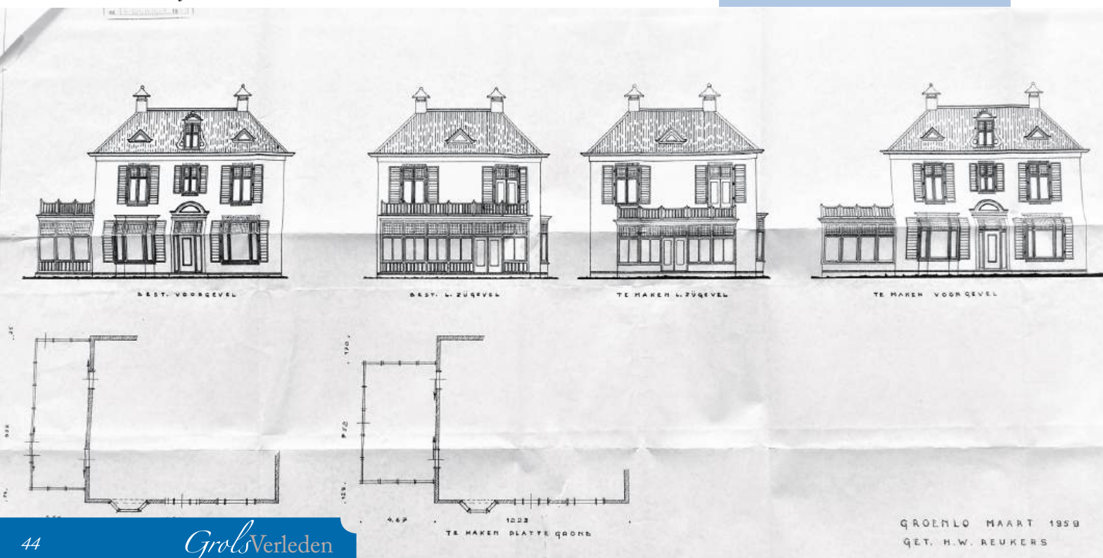
Bouwtekening verbouwing serre 1959 (bron ECAL)
