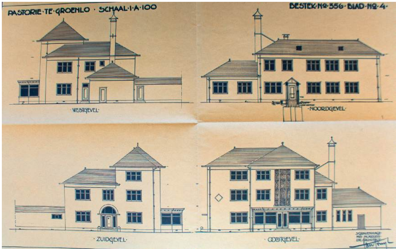
Ontwerp gevels (bron ECAL).
