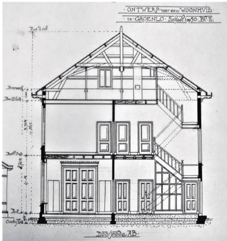
Ontwerp doorsnede (bron NAI toegang STUY-129)
