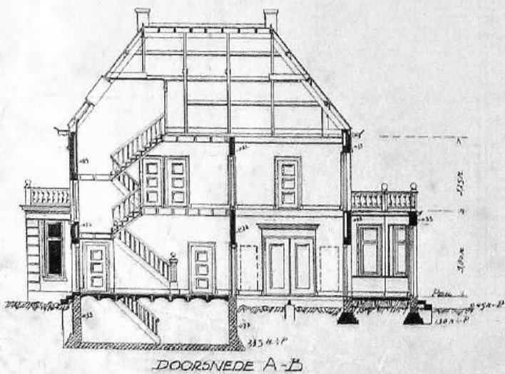
Ontwerp woonhuis door Stuyt en Wiegerinck (bron NAI toegang STUY-130)
