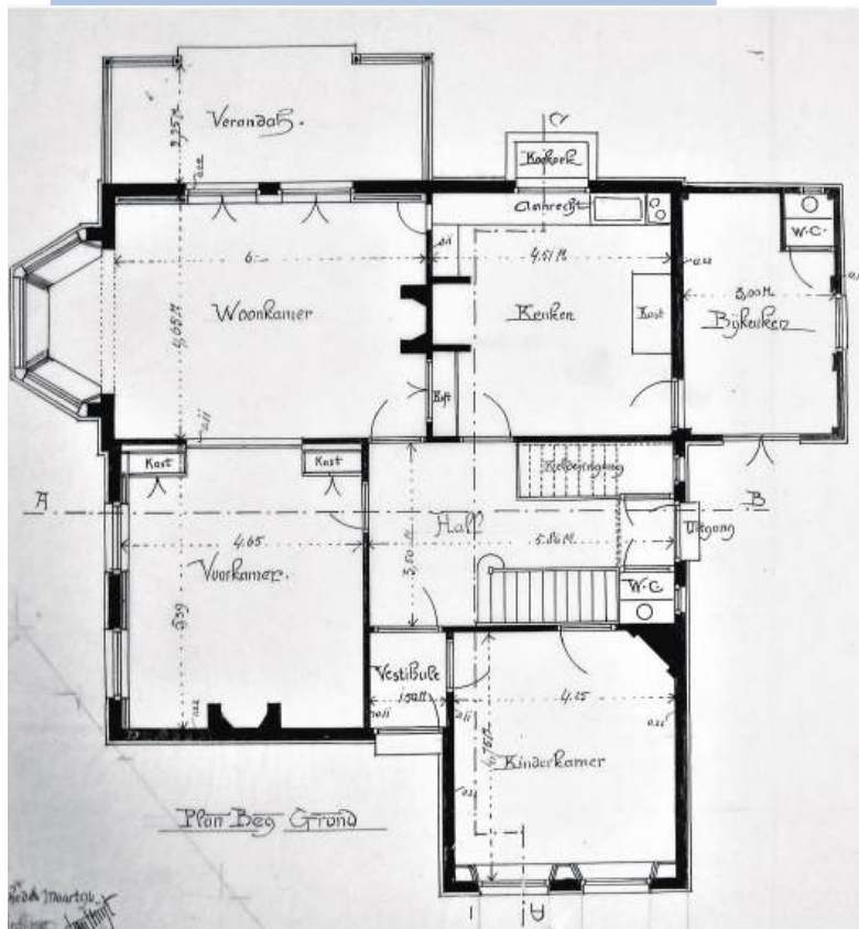
Ontwerp plattegrond (bron NAI toegang STUY-129)
